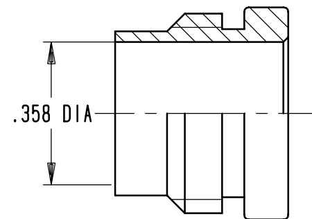
CLAMP NUT
